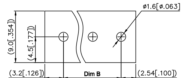
P.C.B LAYOUT
