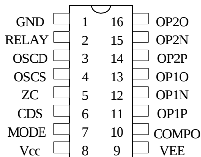
PT8A2648P/2648W
