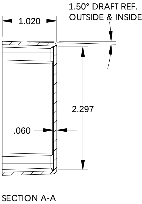
SECTION A-A
