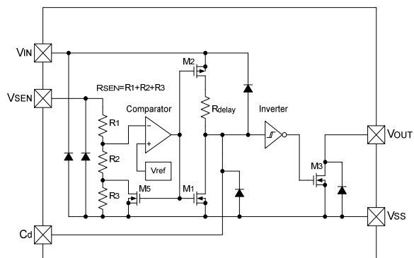
(4) XC6118NxxB
