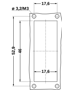
Panel cutout: VS-15-A
