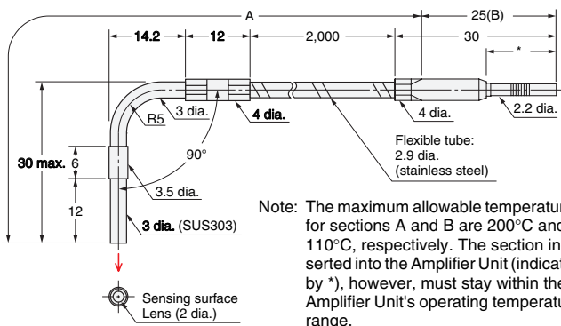
E32-T84S-S (R25)
