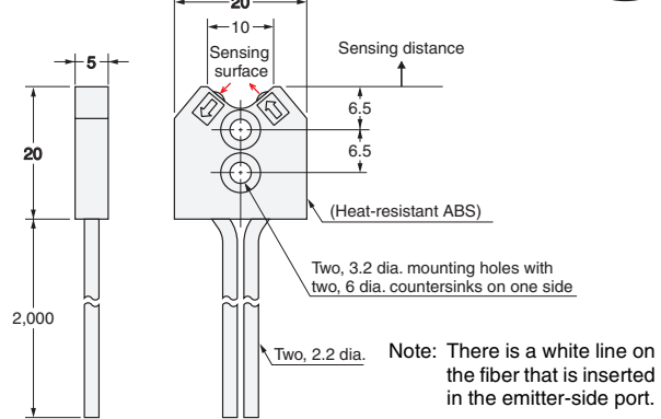
E32-L25A R25
