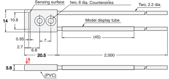
E32-L25L R10
