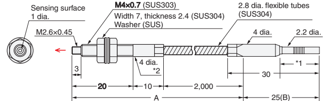
E32-T61-S (R25)
