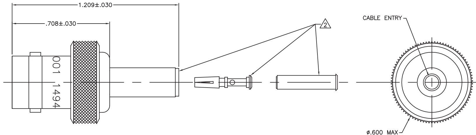
UCJ220-001 SHOWN
