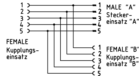
WIRING DIAGRAM Verdrahtungsplan
