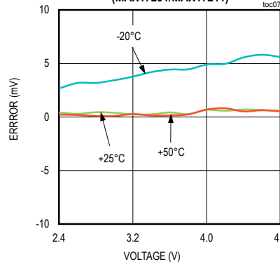
CELL1 VOLTAGE ADC ERROR (MAX17201/MAX17211) toc07
