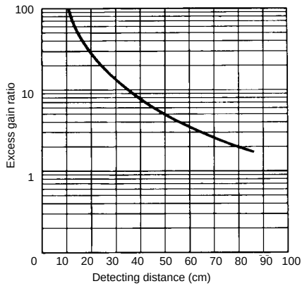
E3C-DS5W
