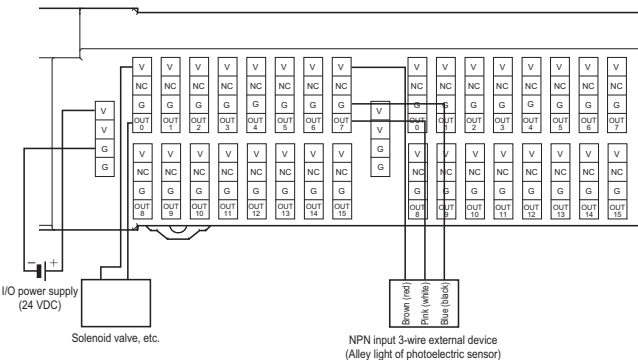
GX-OD3218 (NPN)
