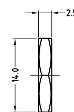
METAL NUT
