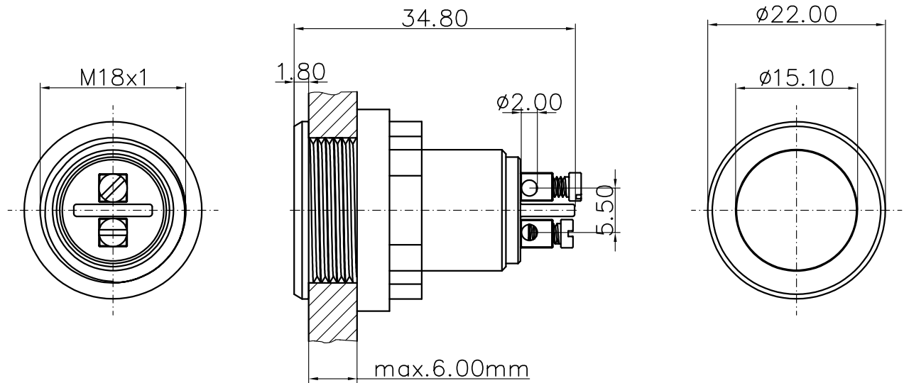
MCS 18 ES
