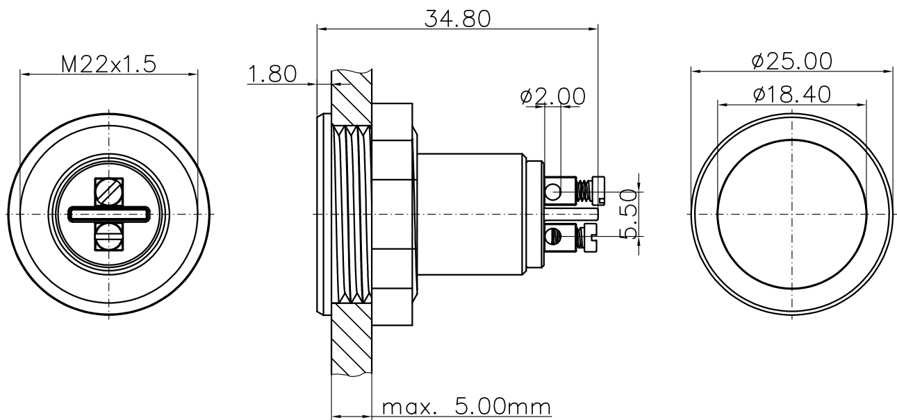
MCS 22 ES
