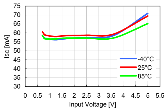
Isc vs VIN
