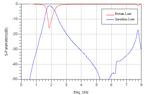
RFBPF1109B201T
