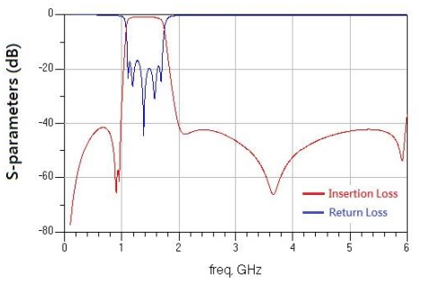
RFBPF1109B101T
