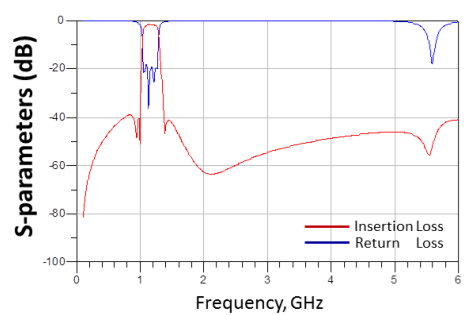
RFBPF1109B201T
