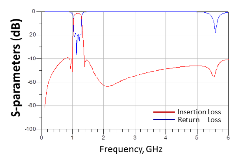
RFBPF1109B201T
