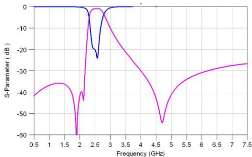
RFBPF2012080AGT
