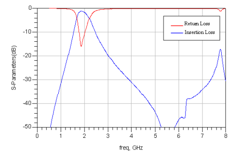
RFBPF1109B201T
