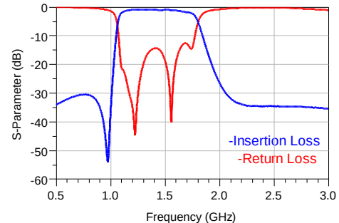
RBBPF3225180C77B1U
