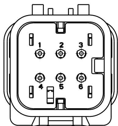
776537-3 SCALE 2:1
