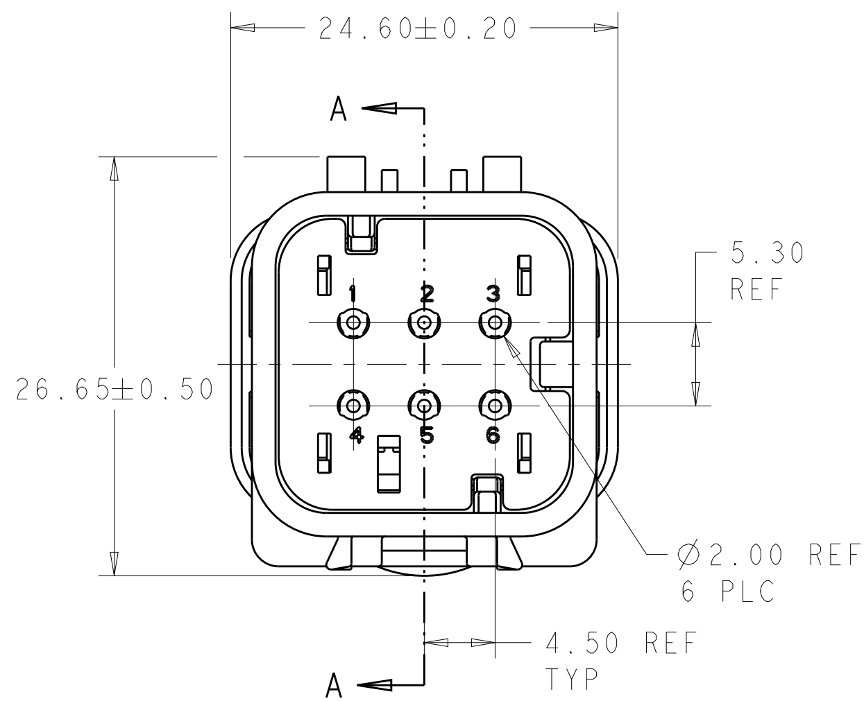
776537-1 SHOWN
