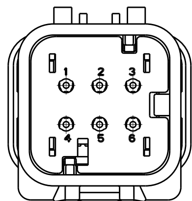
776537-2 SCALE 2:1
