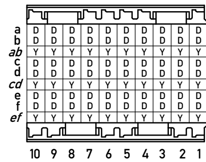
Lochbild für Leiterplatte (Bestückungsseite)
