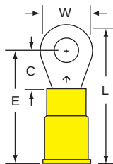
13-8-NB Stud Size 8 Wire Range 12-10
