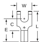
BS-22-8 Stud Size 8 Wire Range 16-14
