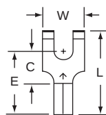
BS-22-6 Stud Size 6 Wire Range 16-14
