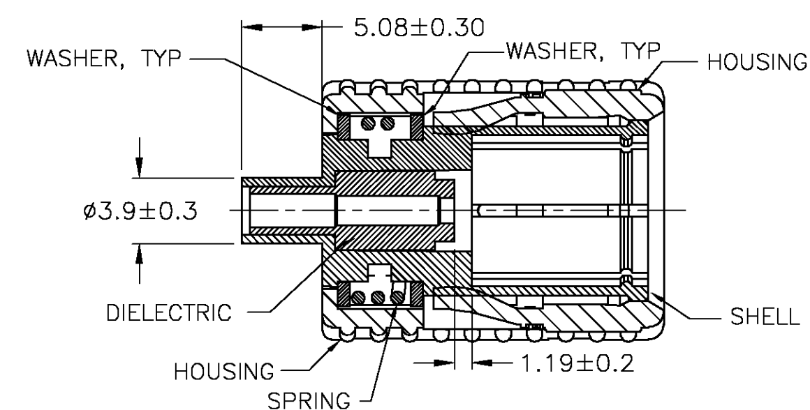
SECTION A-A 109763-3
