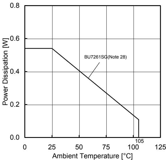
(d)BU7261SG
