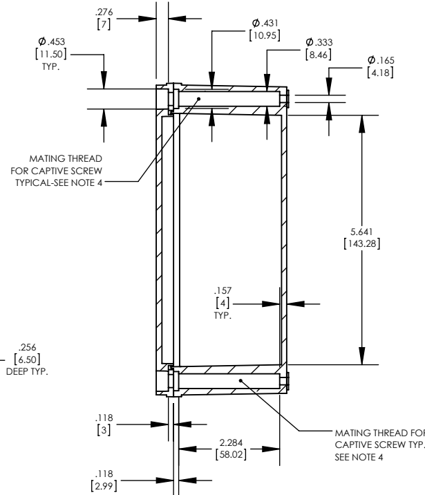
SECTION D-D
