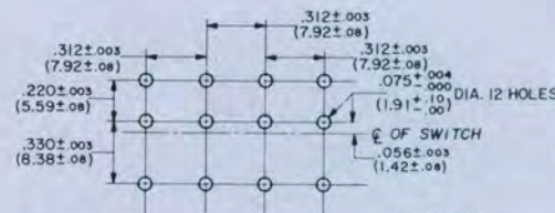
P.C. LAYOUT
