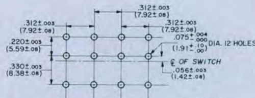
P.C. LAYOUT
