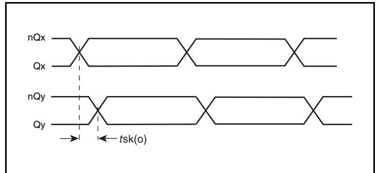
Output Skew
