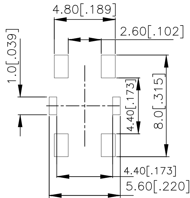
P.C.B. LAYOUT
