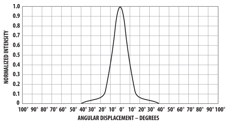
Figure 8. HLMP-Q106/-Q156.
