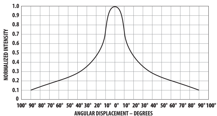
Figure 9. HLMP-Q102/-Q152
