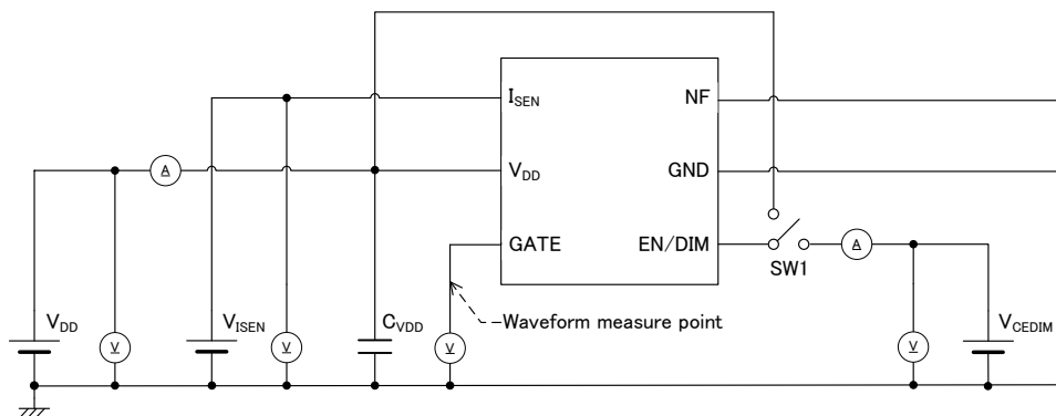
2) CIRCUIT②
