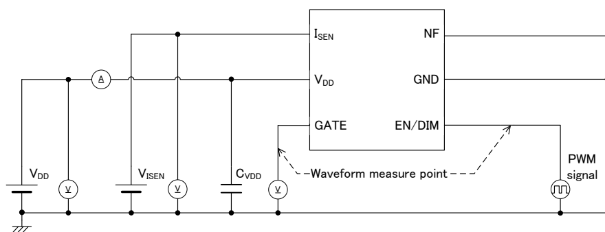
3) CIRCUIT③
