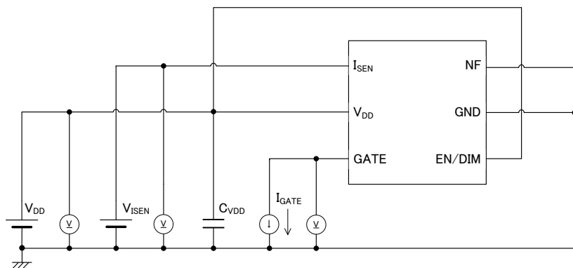
3) CIRCUIT③
