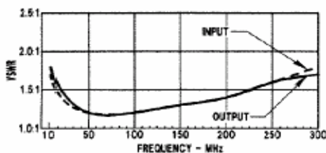
Input/Output VSWR
