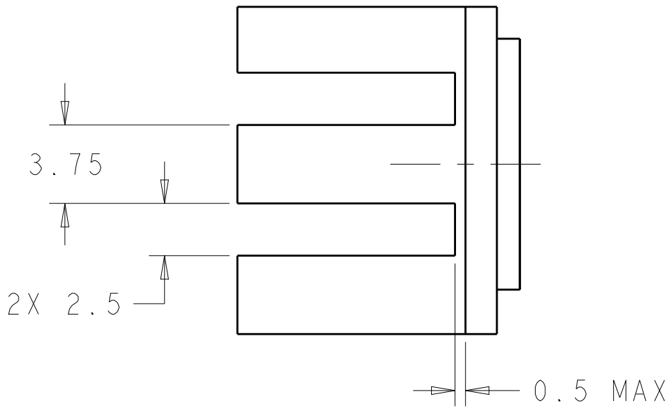
2170394-7/9 SCALE 4:1
