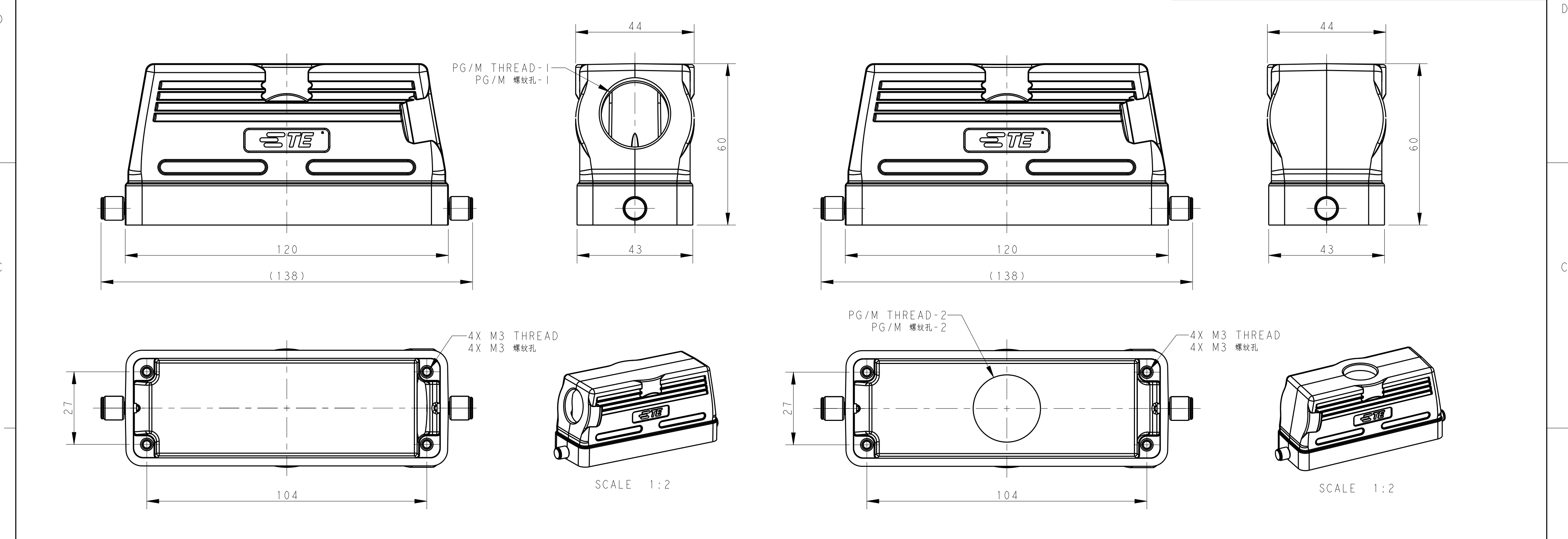
TYPE 1: LOW CONSTRUCTION, SIDE ENTRY 类型1: 低结构, 侧出 TYPE 2: LOW CONSTRUCTION, TOP ENTRY 类型2: 低结构, 高出
