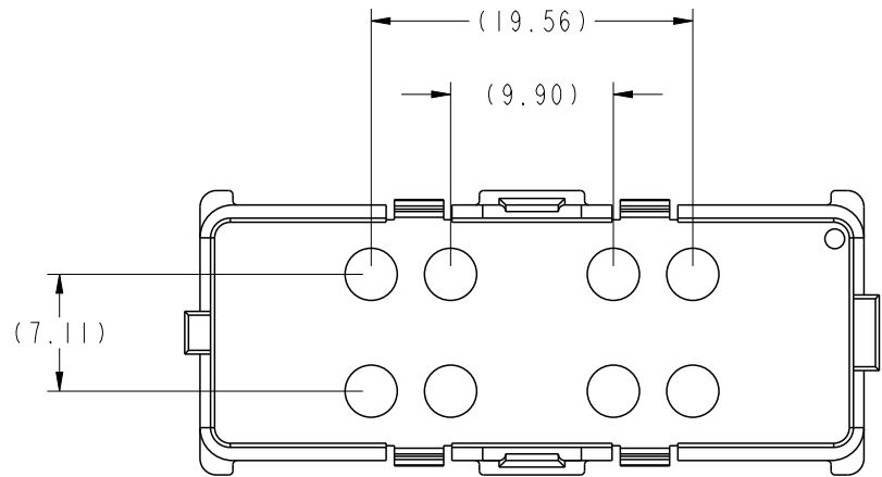
84504-002 SHOWN SCALE 2:1
