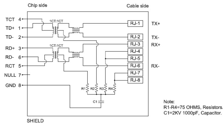
009 (100 Base-T)
