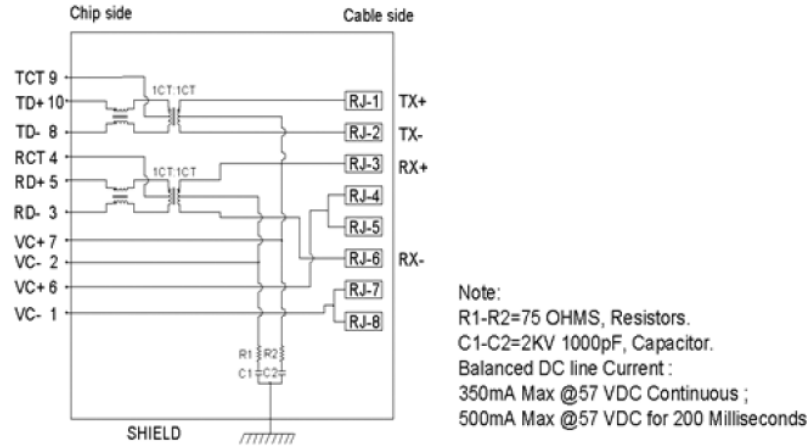
114 (100 Base-T & PoE)
