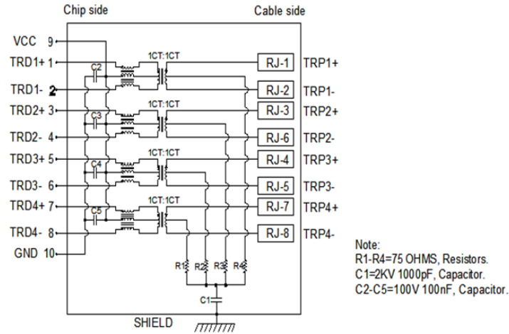
805 (2.5G Base-T)
