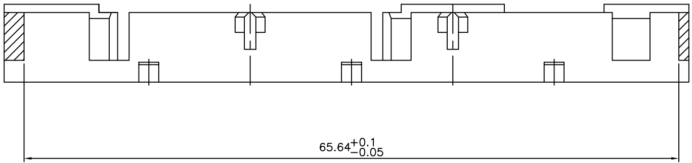
SECTION A-A
