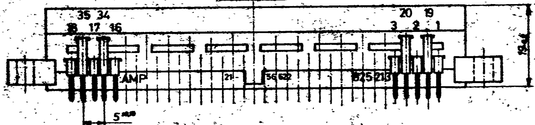
Ansicht "X"
