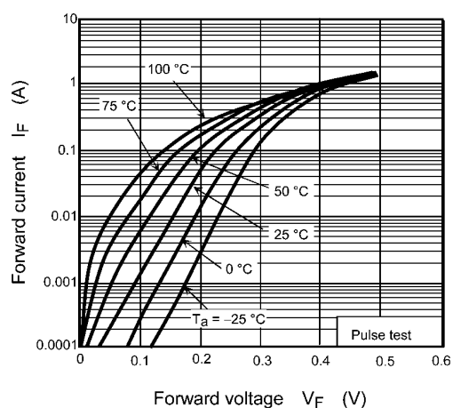
Fig. 9.1 I_F - V_F
