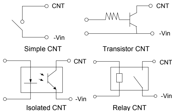
Fig. 71 CNT circuits
