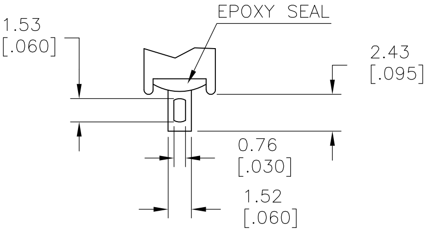
SOLDER LUG
