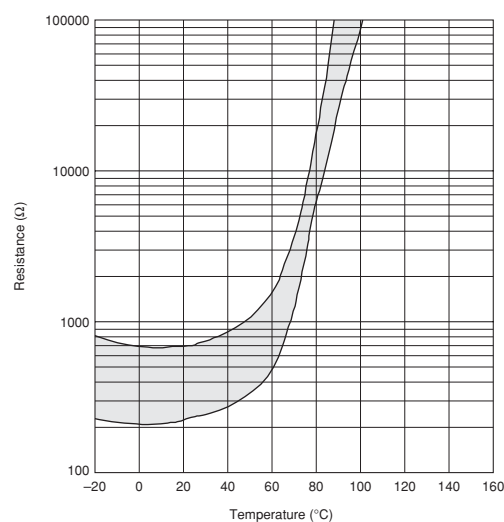
PRF18BF471RB5RB
