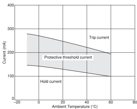
PTGL09AR390N0B52A0
