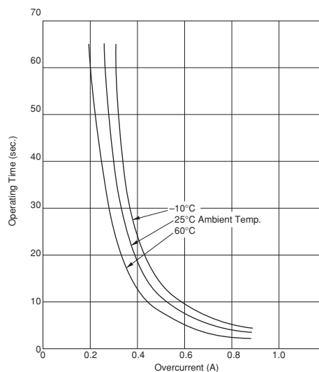
PTGL09AR250H8B52B0
