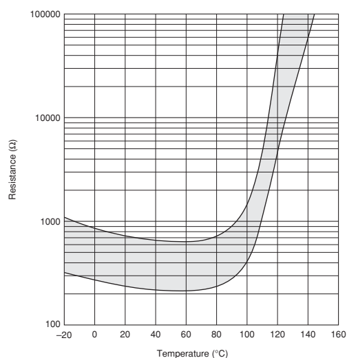
PRF18/21BB471Q Type
