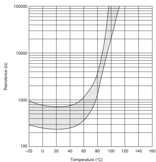
PRF18BE471RB5RB
