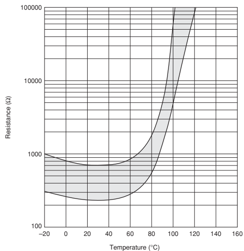
PRF18/21BD471Q Type
