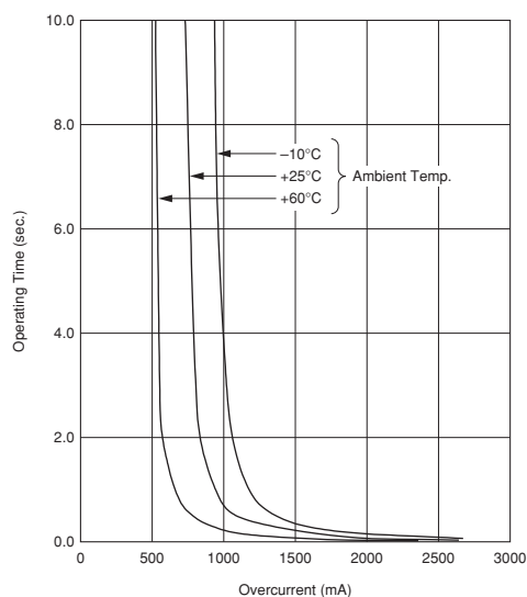
PRG21BC0R6MM1RA
