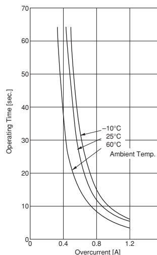
PTGL12AR150H8B72B0
