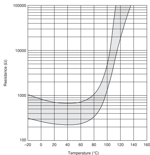
PRF18/21BC471Q Type
