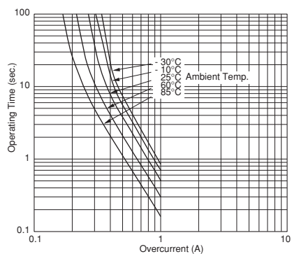
PTGL04AS100K3B51B0
