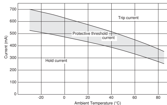
PTGL09AS3R3K4B51B0
