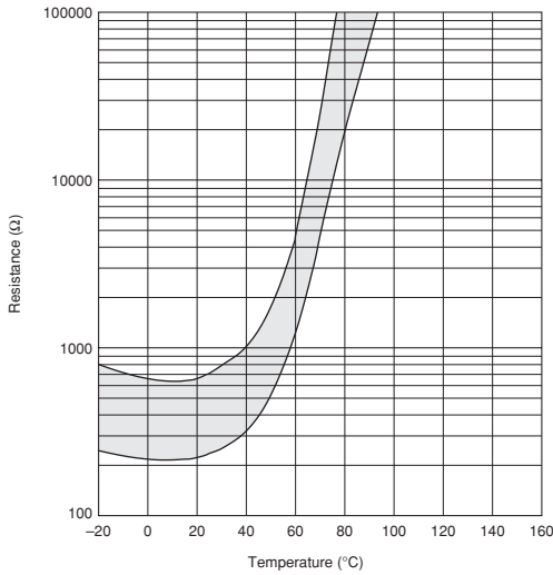
PRF18BG471Q Type
