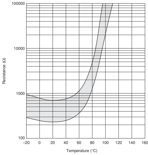
PRF18/21BE471Q Type
