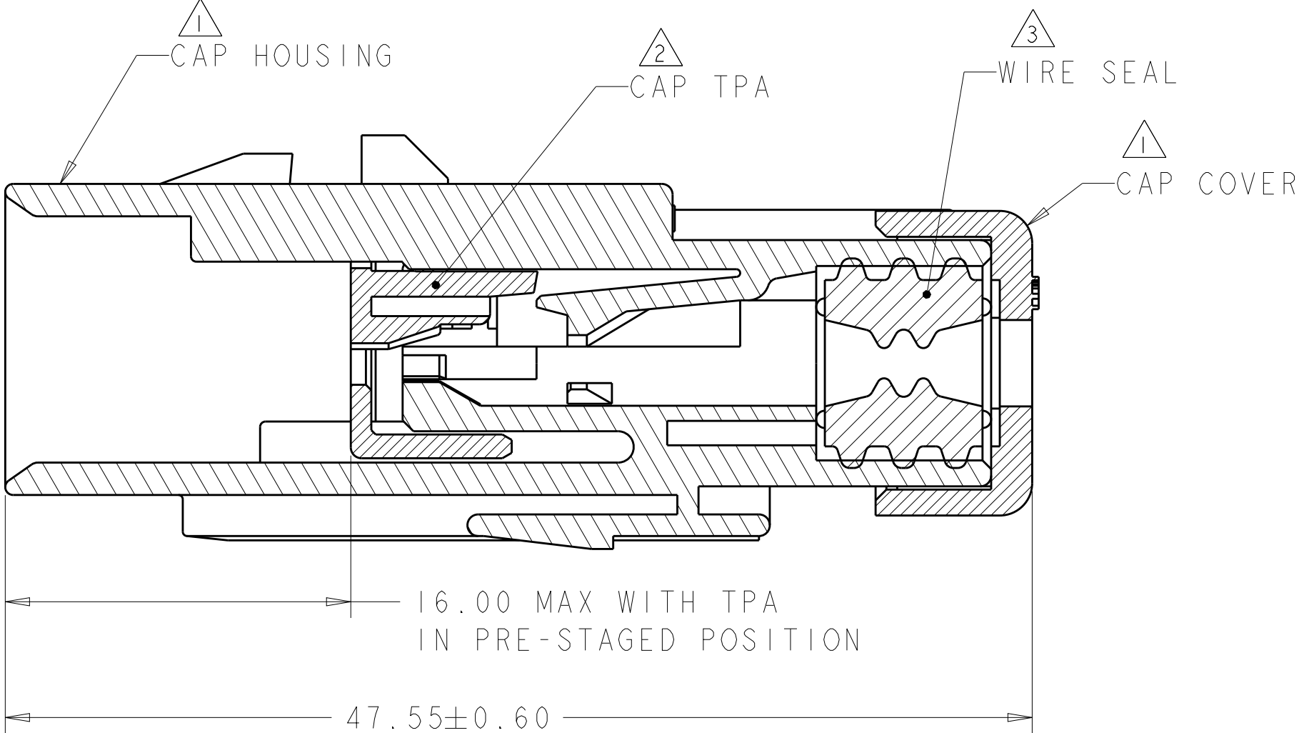
SECTION A-A
