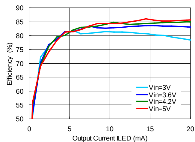
5LED, L=22\mu H (LQH32CN220K53)
