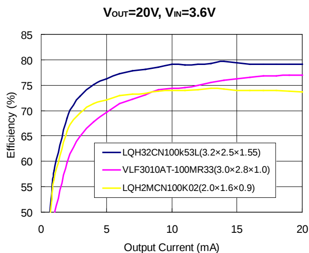
4LED, L=10\mu H (LQH32CN100K53)
