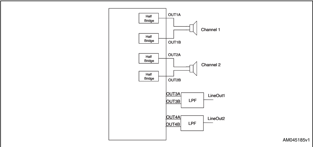
Figure 23. OCFG = 00 (default value)
