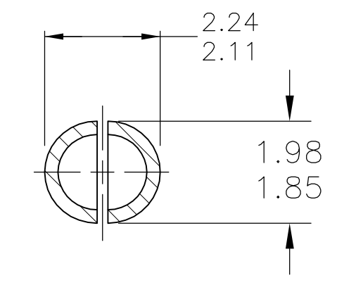
SECTION A-A SCALE 10:1
