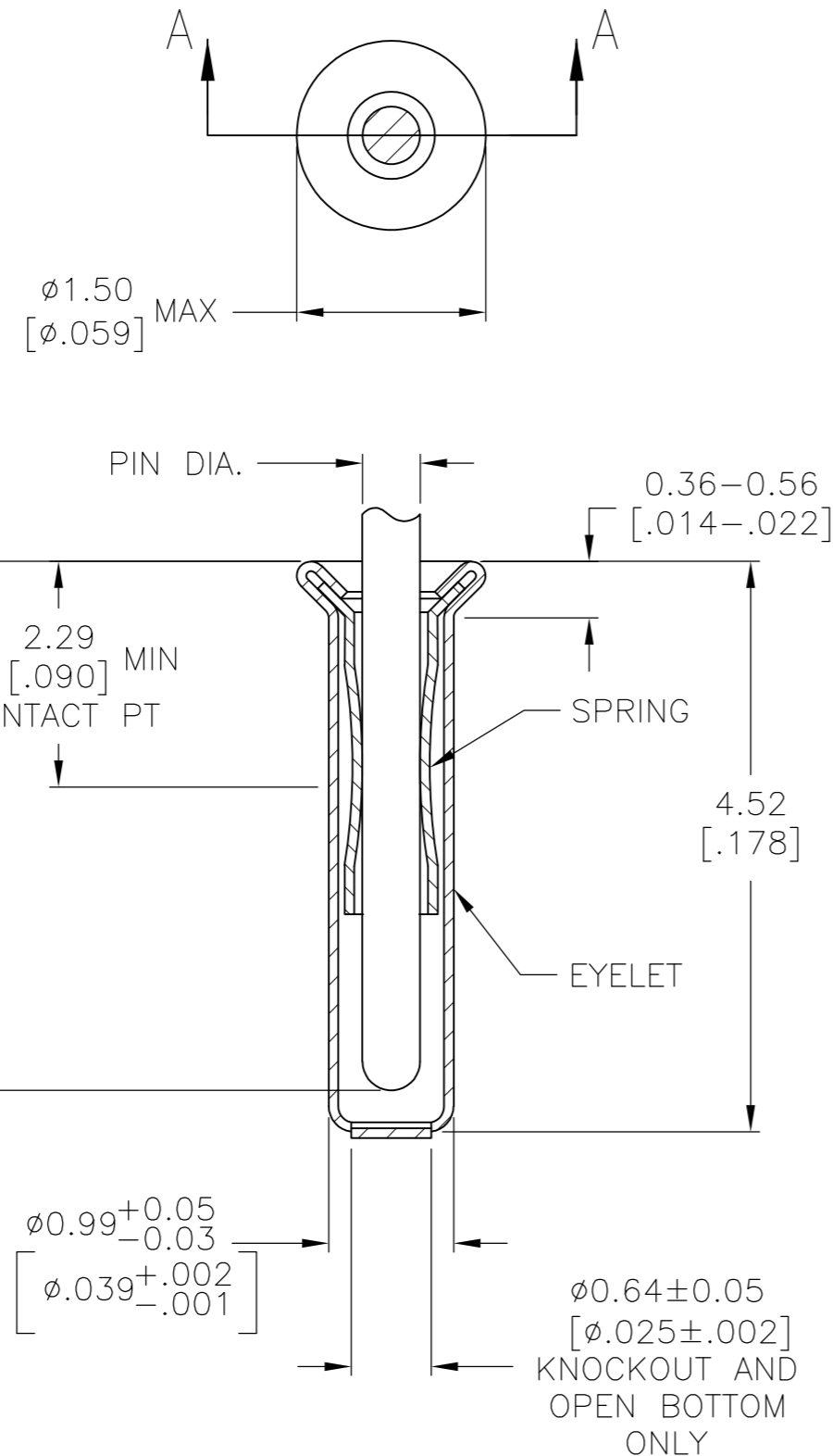
SECTION A-A
