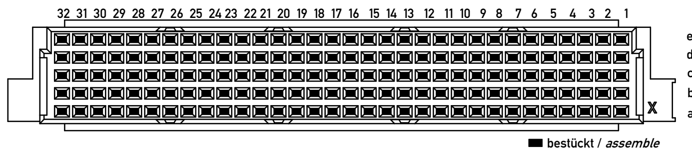
Bestückungsplan / contact layout
