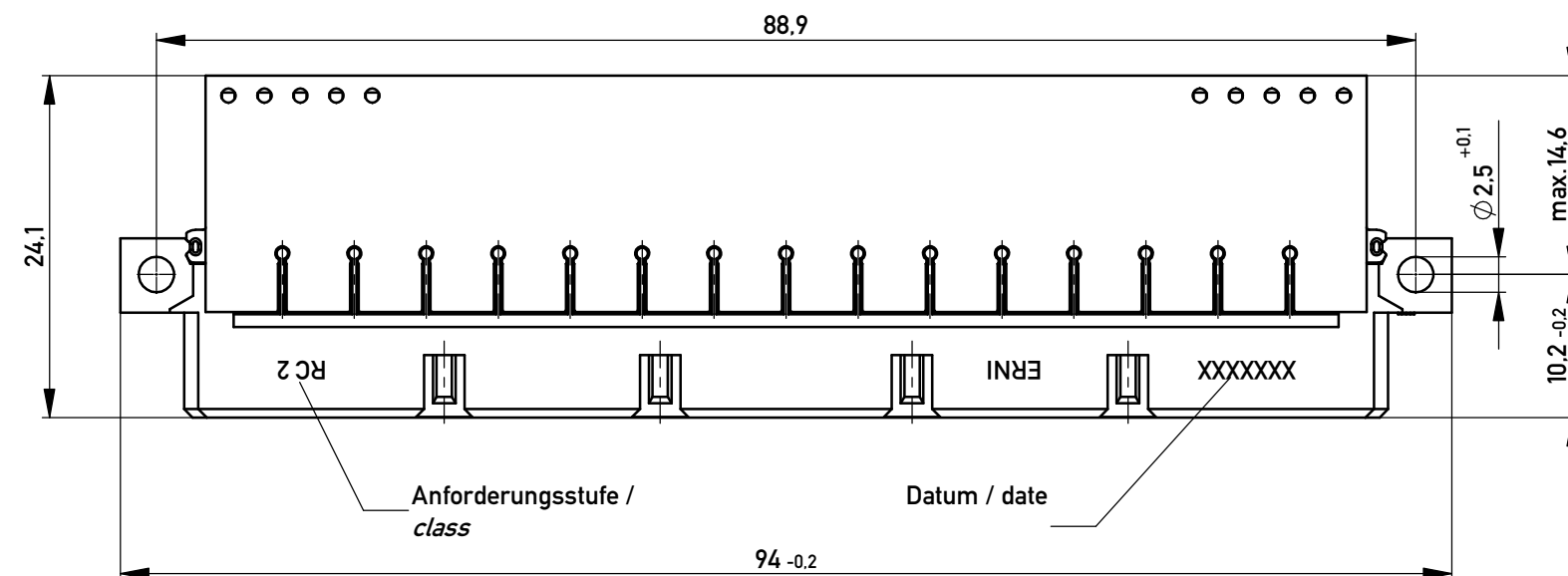
Bestückungsplan / contact layout
