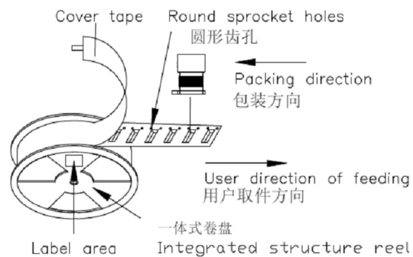
TAPE&REEL示意图
