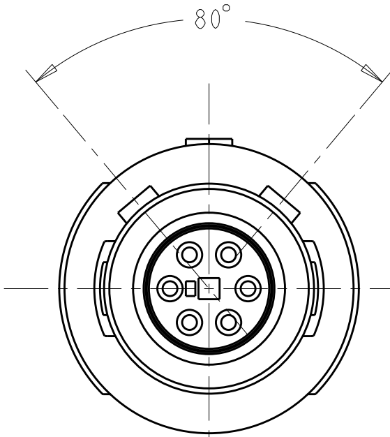
80° KEYING SCALE 4:1
