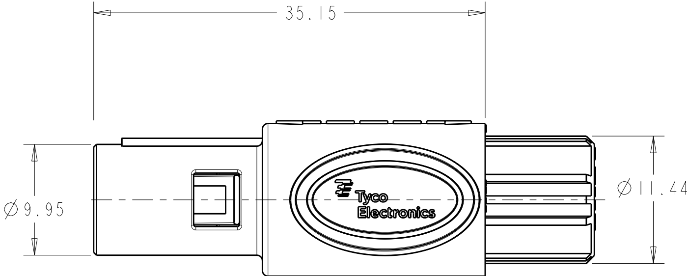
SCALE 3:1
