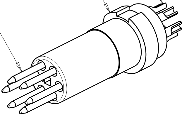
INSERT SUB-ASSY
