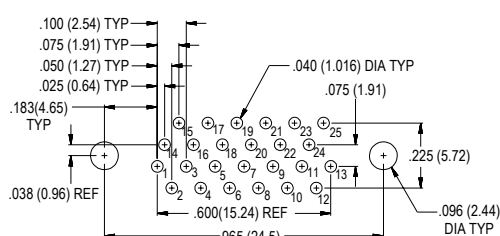
25 Socket MWDM-25SCBS
